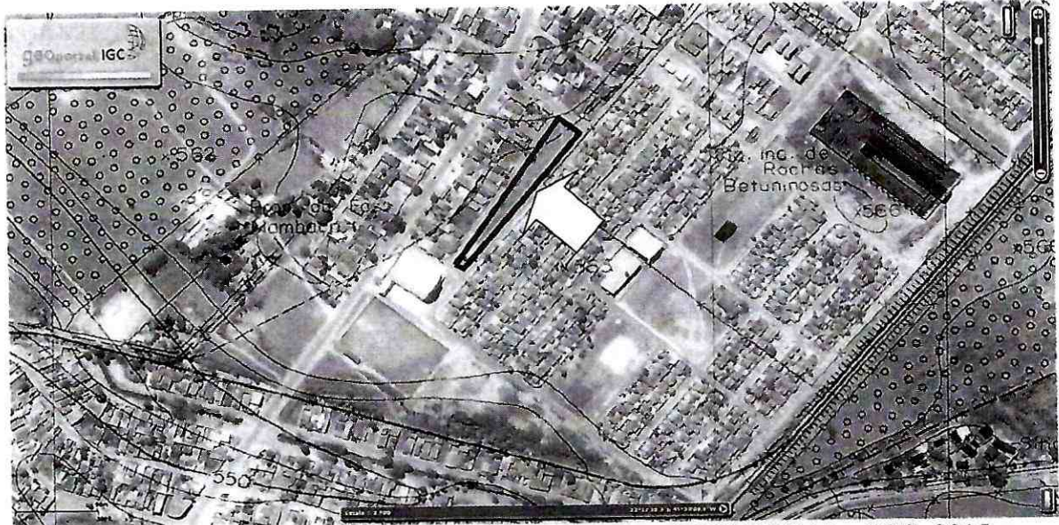
Imagem 01 – Localização da área solicitada. Fonte: GEOPORTAL – IGC, 2015.
