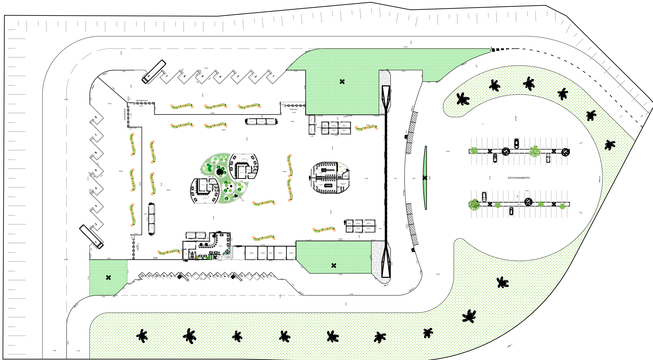
PLANTA BAIXA - IMPLANTAÇÃO ESC. 1:1000
